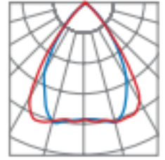
Reflector 50°
