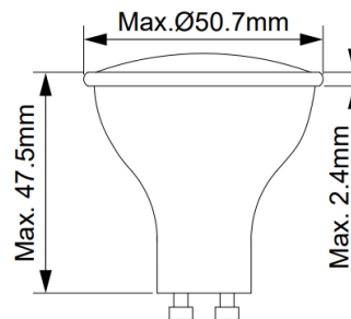
GU10 Ø51(IEC 60357)
