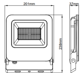
VEN50-SCT
