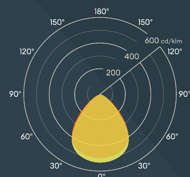
Ø260mm HBASIV40
